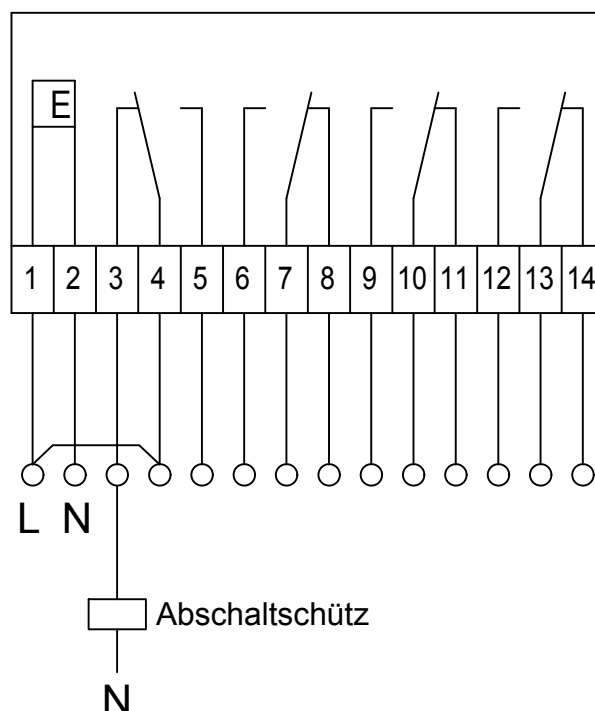
Tonfrequenz-Rundsteuerempfänger
