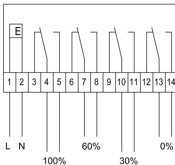
Funk-Rundsteuerempfänger
