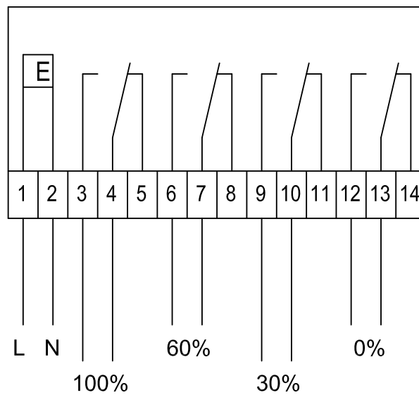
Tonfrequenz-Rundsteuerempfänger
